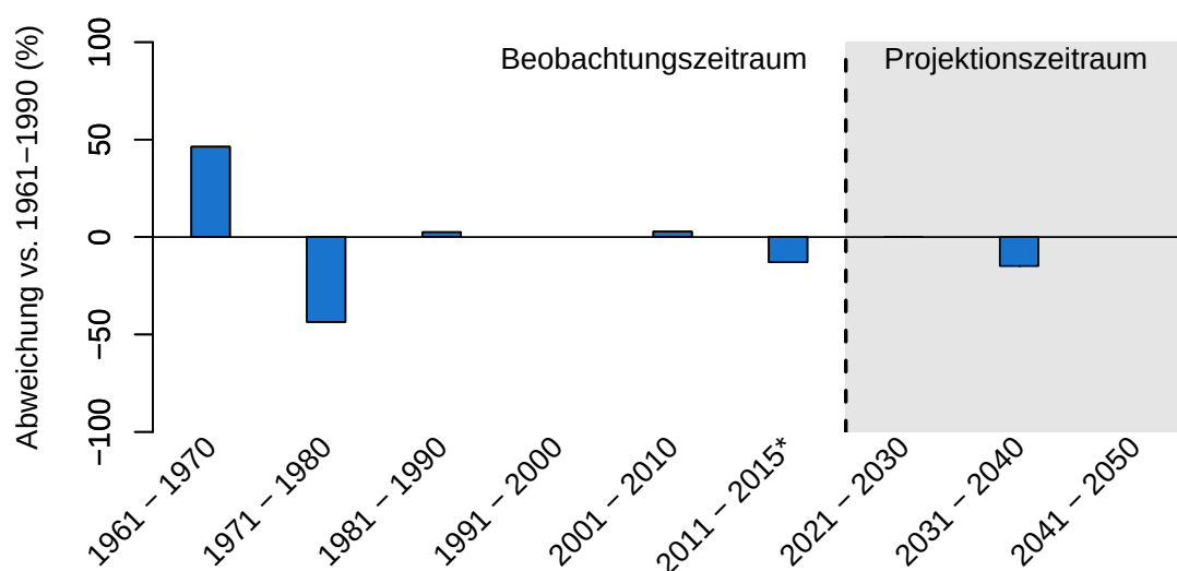
Abbildung 3: Abweichung von Tagen in einem 7tägigen Zeitraum mit einer Schneehöhe größer 20 cm (Referenz 1961–1990) im Gesamtwinter (Dezember–März). Im Projektionszeitraum wird neben dem Mittelwert (farbiger Balken) zusätzlich mit dem Entwicklungskorridor (senkrechte schwarze Linie) die mögliche Bandbreite der Entwicklung angegeben. * Zeitraum entspricht keiner vollen Dekade.
